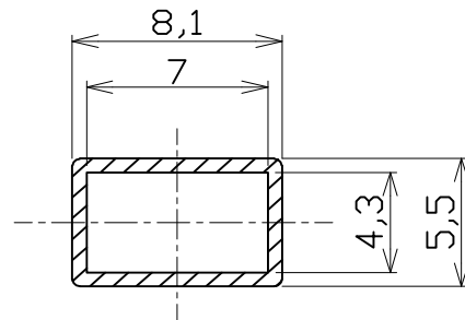
SEC A-A
